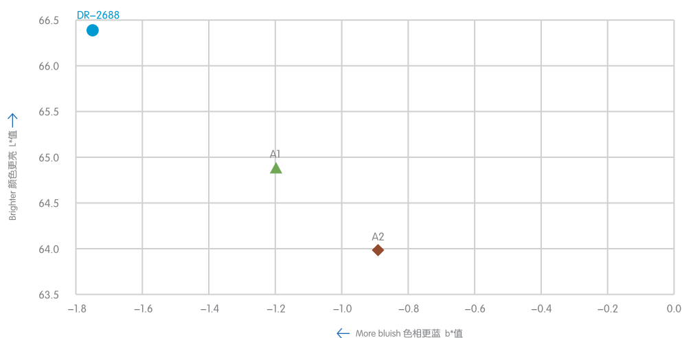
Undertone and tinting strength in grey PVC-P ( \text{TiO}_2 content: 4PHR) 在聚氯乙烯体系PVC-P (灰色) 中的底相和着色力 (钛白粉含量4PHR) (HG/T 4769.3-2014)
